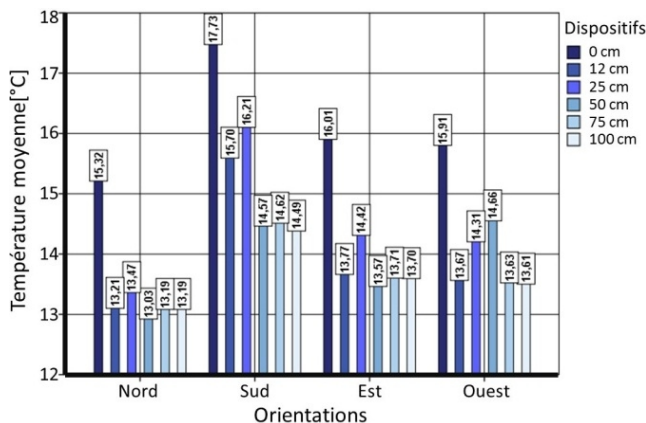
Fig. 6. Températures moyennes de la période hivernale.
